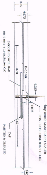
ขยายรอยต่อ CONSTRUCTION JOINT
